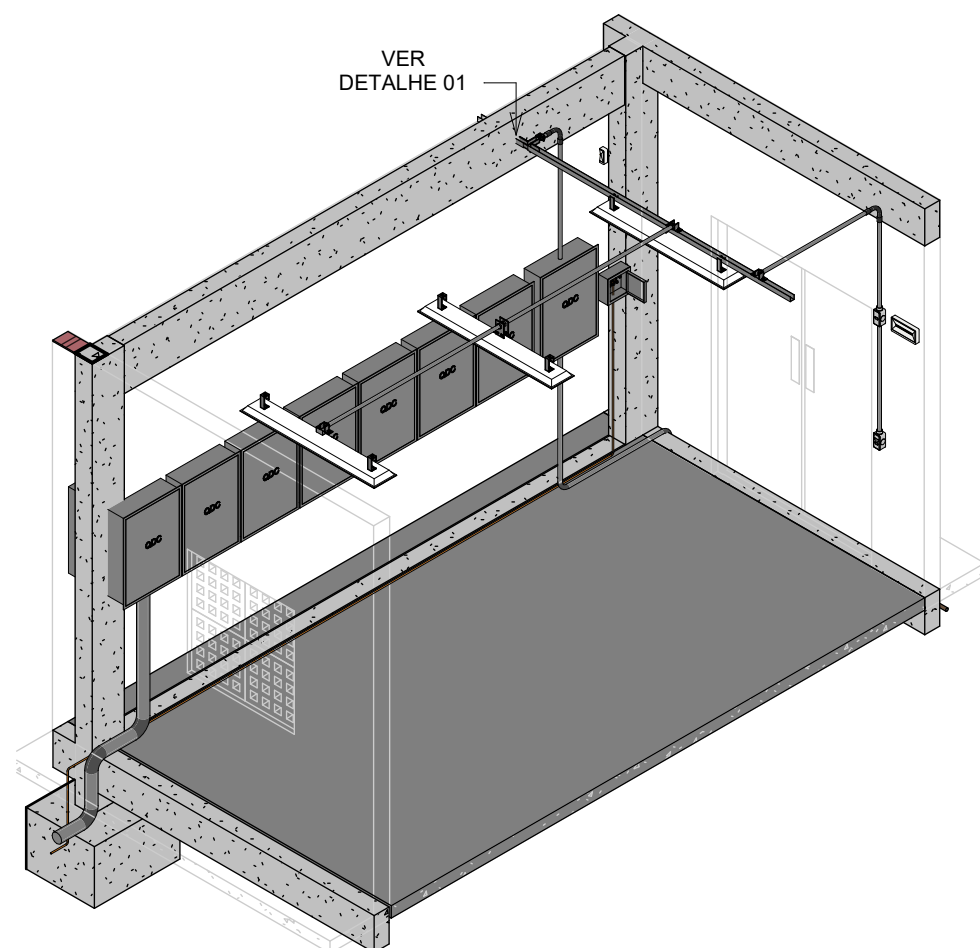
ISOMÉTRICO - SALA DE COMANDO ESC.: 1:50
