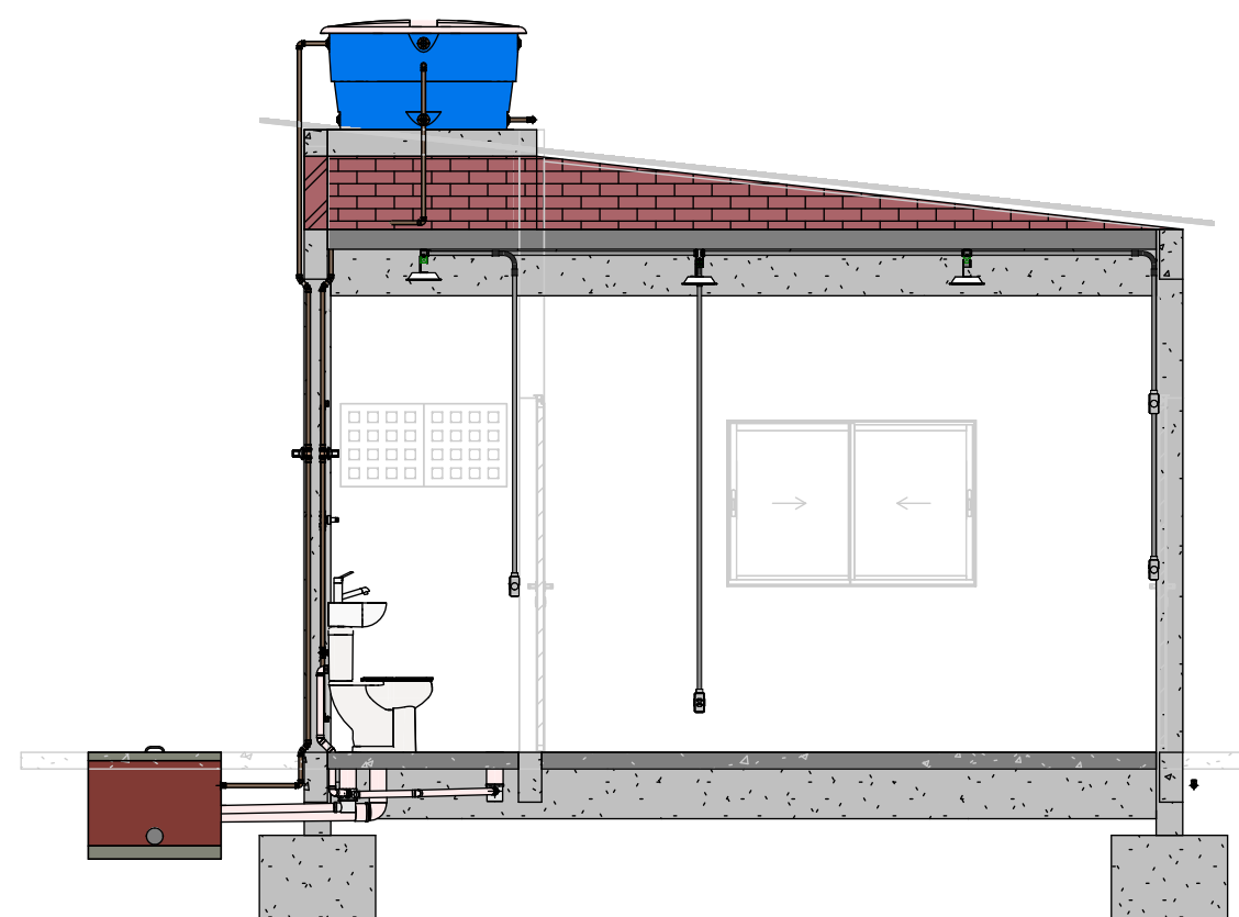
CORTE - SALA DO OPERADOR + BANHEIRO ESC.: 1:50
