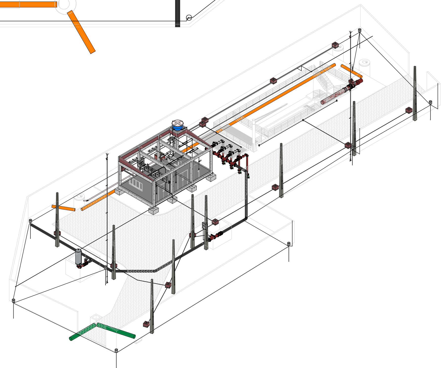
ISOMÉTRICO - EEE DEFINITIVA CEREJEIRAS ESC.: 1:50
