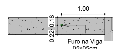
DETALHE 01 ESC.: 1:50
