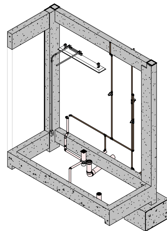
ISOMÉTRICO - BANHEIRO ESC.: 1:50
