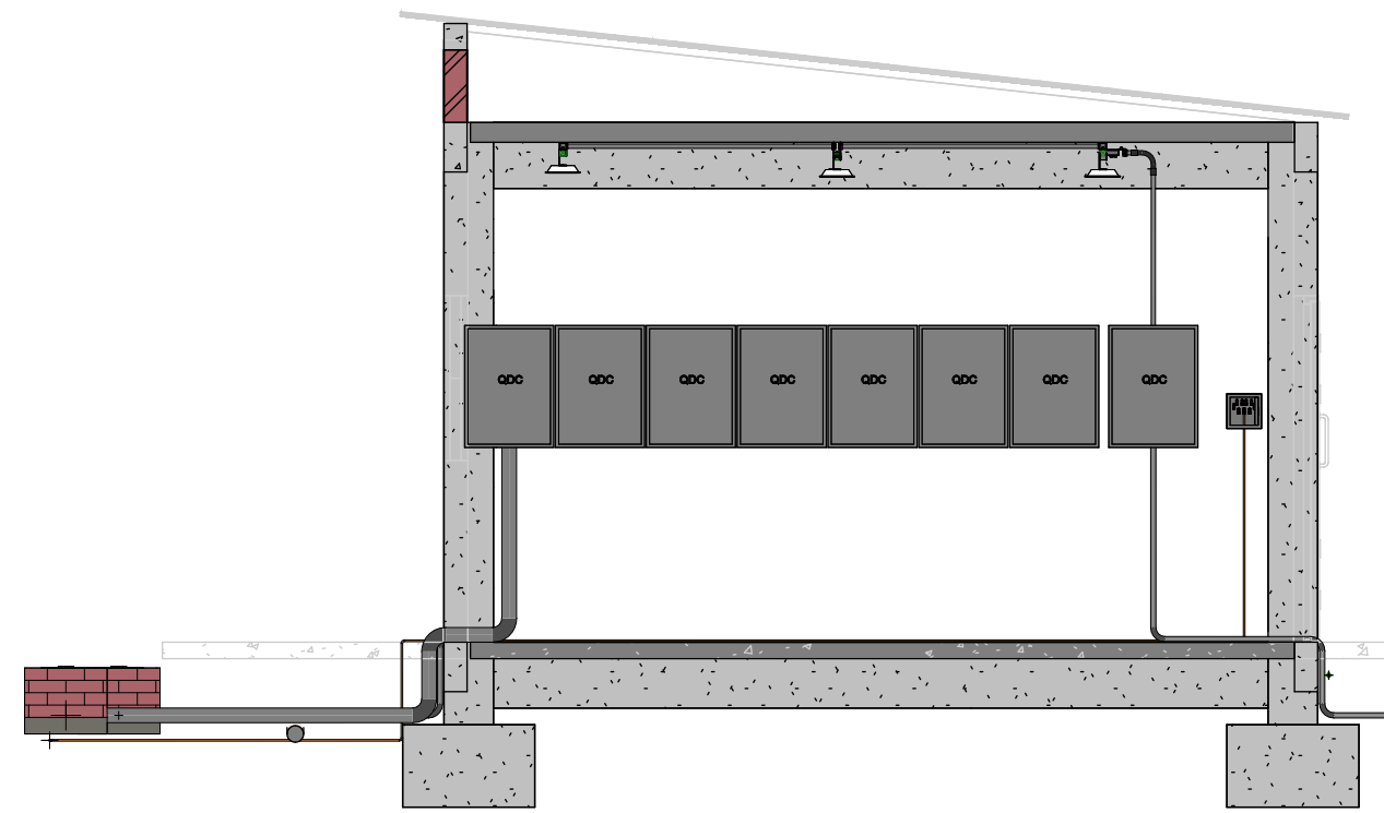
CORTE - SALA DE COMANDO ESC.: 1:50
