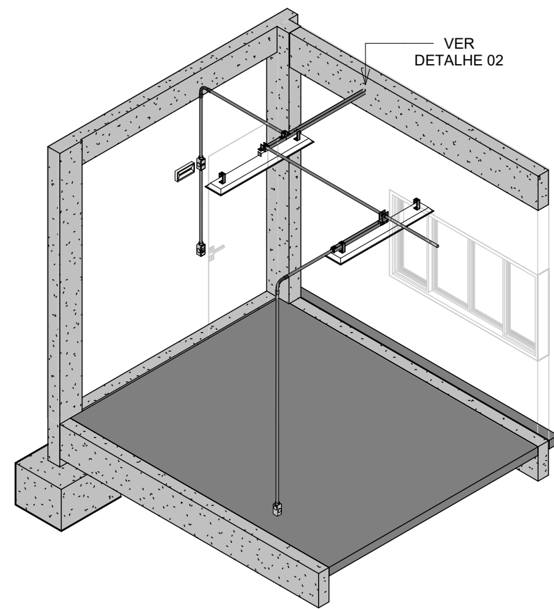
ISOMÉTRICO - SALA DO OPERADOR ESC.: 1:50
