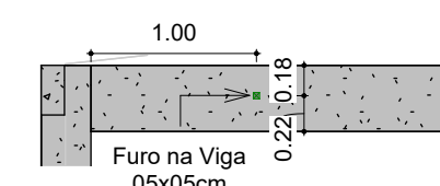
DETALHE 02 ESC.: 1:50
